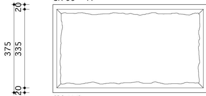
(製品図)
