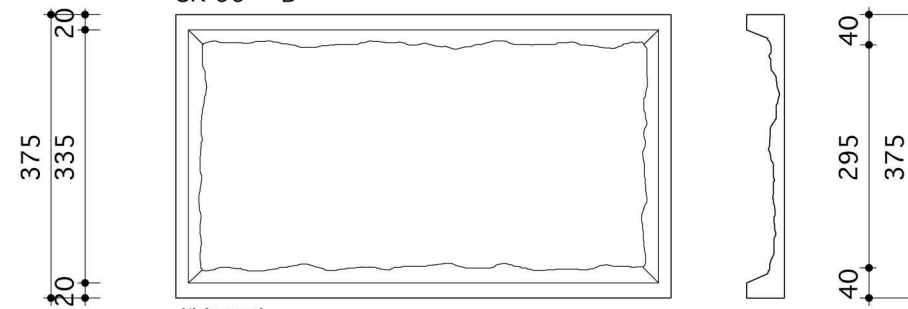
(製品図)
